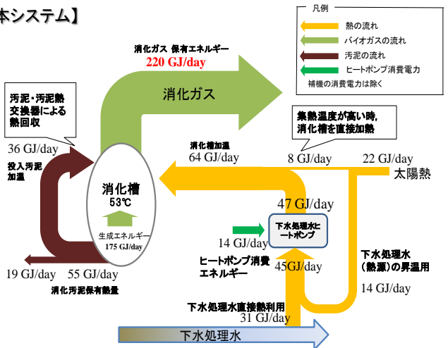
図3 本システムを導入した下水処理場のエネルギーフロー例
