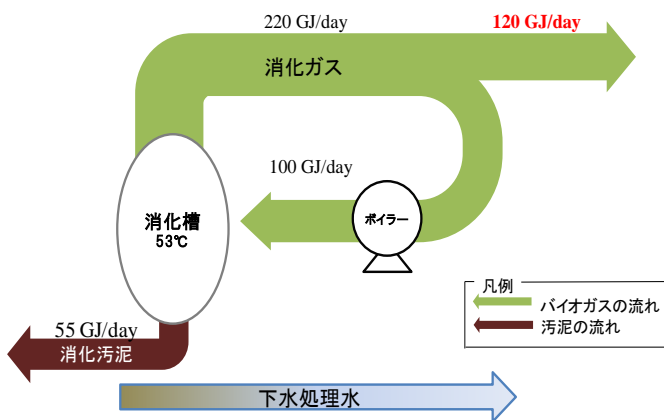
図2 現状の下水処理場のエネルギーフロー
